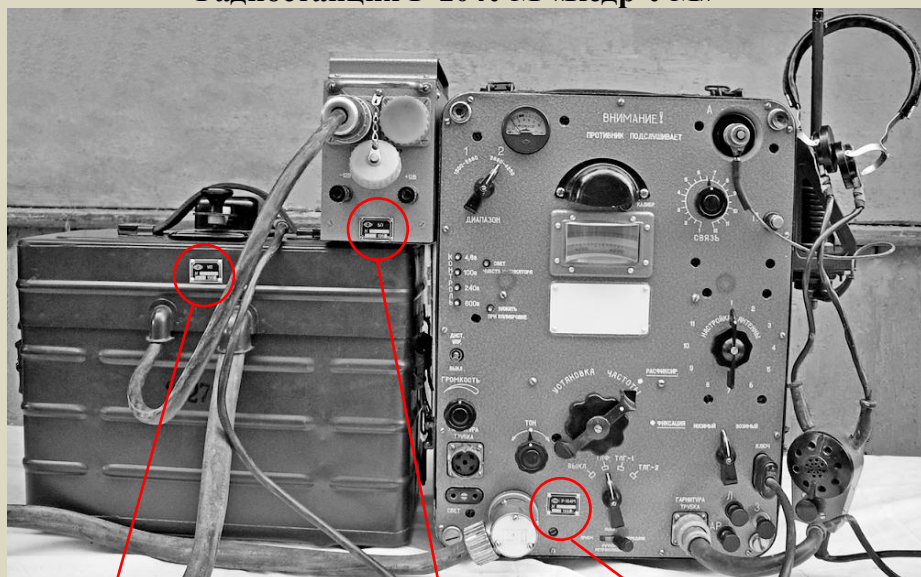
Радиостанция Р-104УМ «Кедр-УМ»
